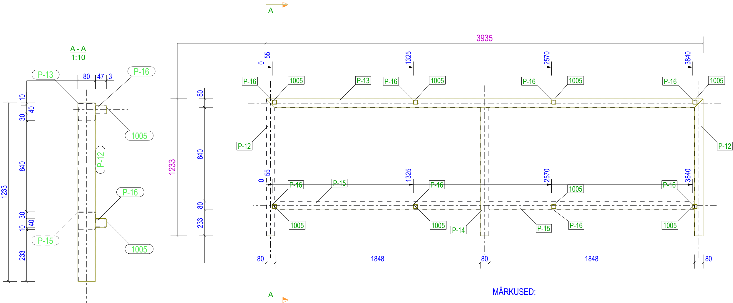
Varikatus VK-1 1:20
